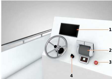
Abb. 48: Bedienelemente
