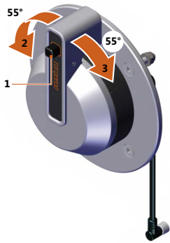
Abb. 89: Bedienung Ferngashebel bei Vorwärts-/Rückwärtsfahrt
