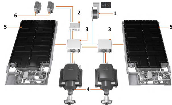
Abb. 49: Komponenten Deep Blue 40i/80i
