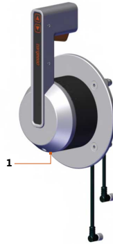
Abb. 64: Ferngashebel – Seitenmontage
